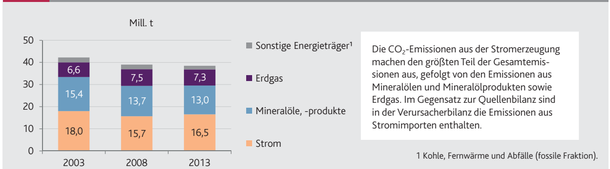
G 11 CO 2 -Emissionen aus dem Endenergieverbrauch (Verursacherbilanz) 2003–2013 nach Energieträgern
