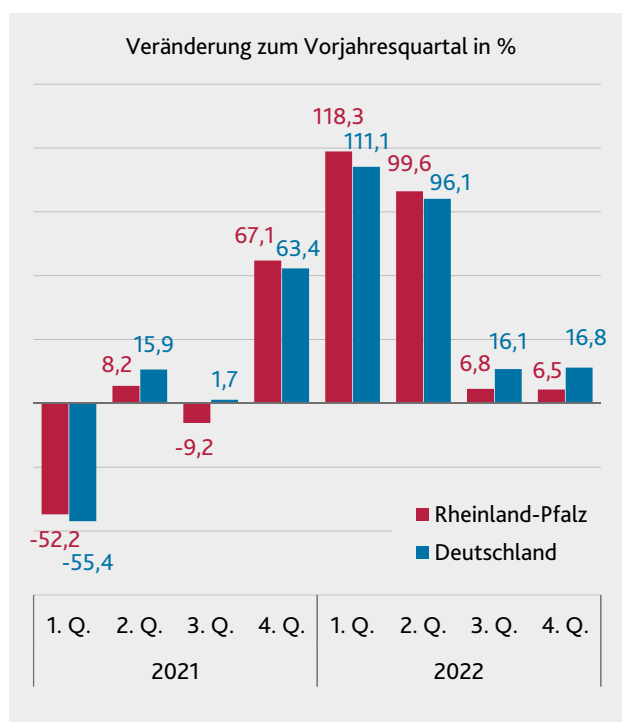
G18 Preisbereinigter Umsatz im Gastgewerbe 2021 und 2022 nach Quartalen
