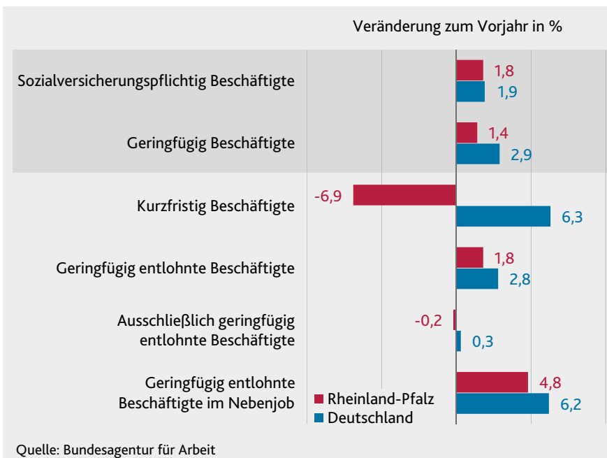
G31 Sozialversicherungspflichtig Beschäftigte und geringfügig Beschäftigte in Rheinland-Pfalz und in Deutschland 2022 nach Beschäftigungsarten
