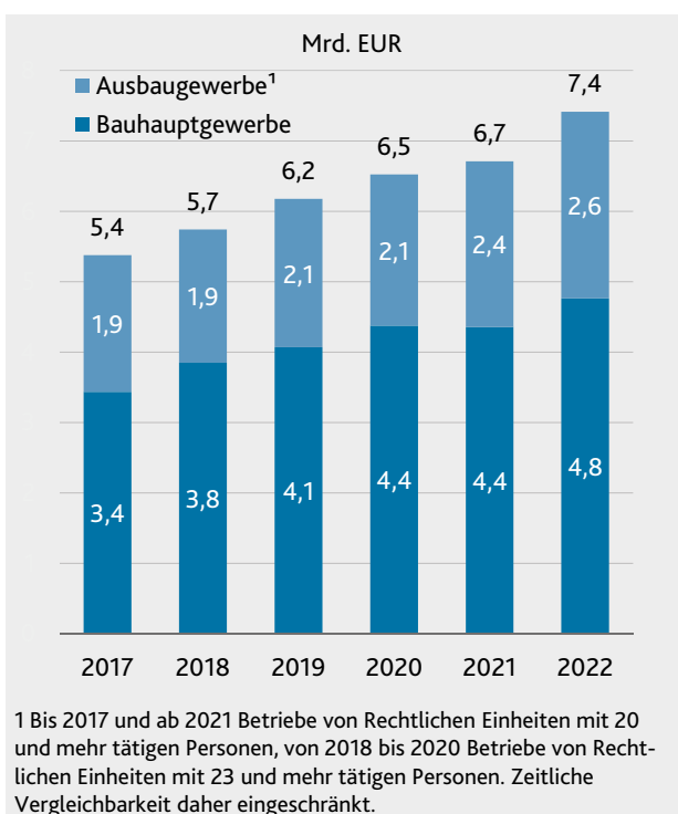
G12 Umsatz im Baugewerbe 2017–2022
