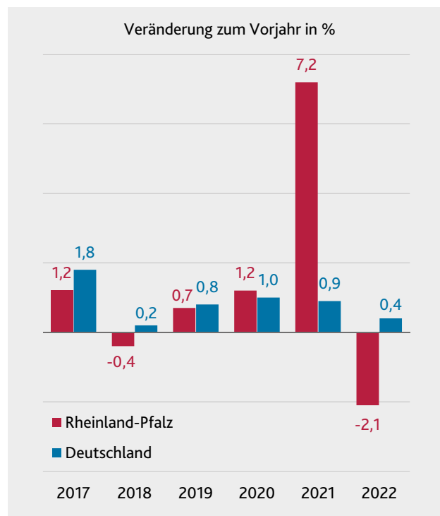
G6 Arbeitsproduktivität (Stundenkonzept) in Rheinland-Pfalz und in Deutschland 2017–2022
