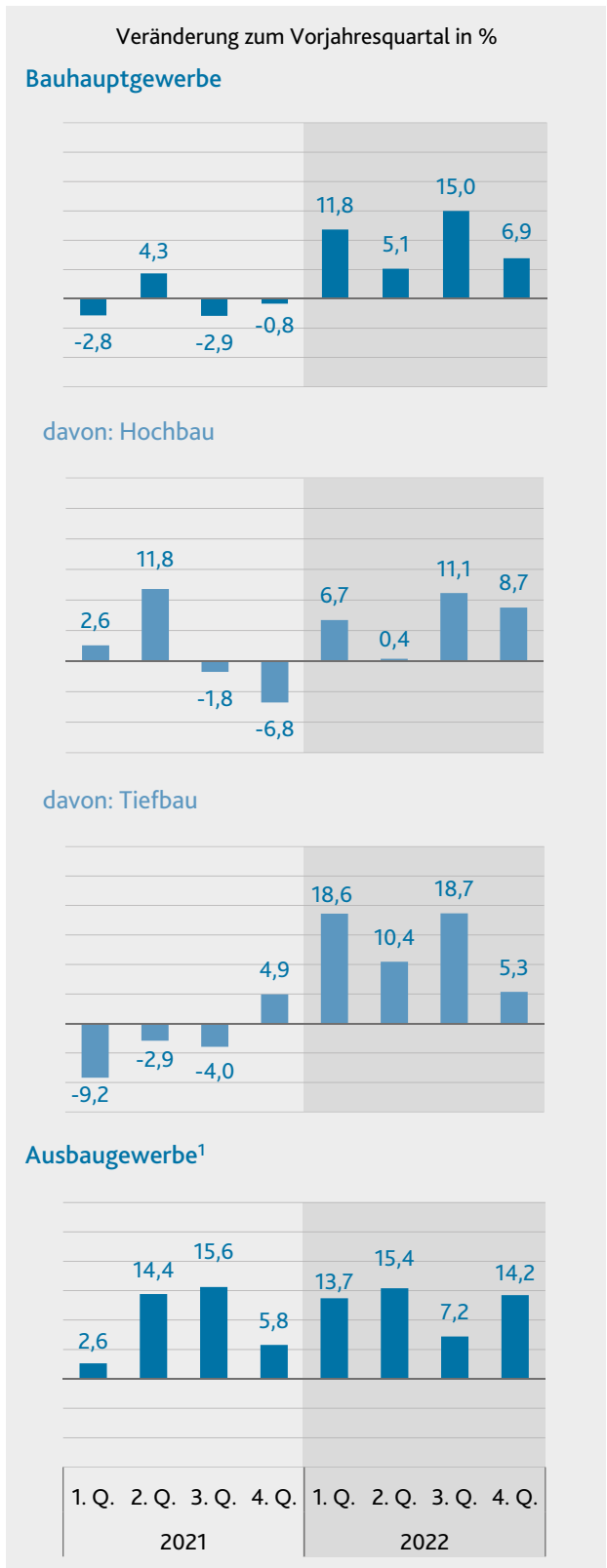
G13 Umsatz im Baugewerbe 2021 und 2022 nach Quartalen
