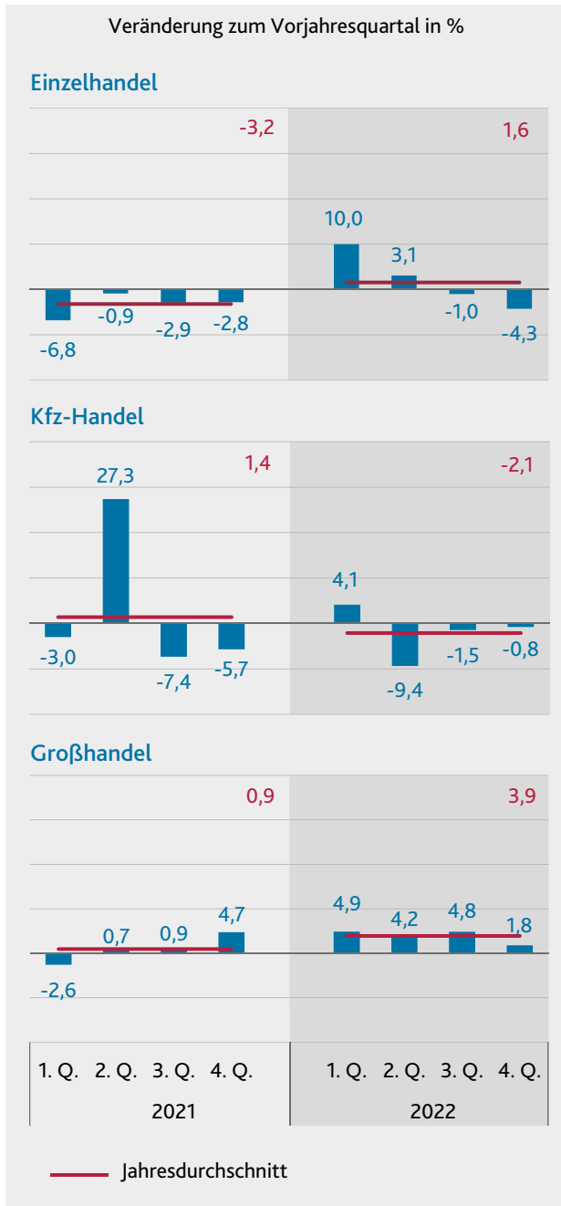
G16 Preisbereinigter Umsatz im Handel 2021 und 2022 nach Quartalen
